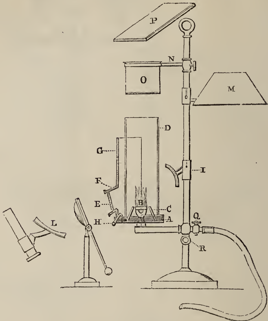
Fig. 48.—Gas-lamp, &c.
