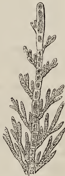
Fig. 123.— Sphacelaria cirrhosa .
