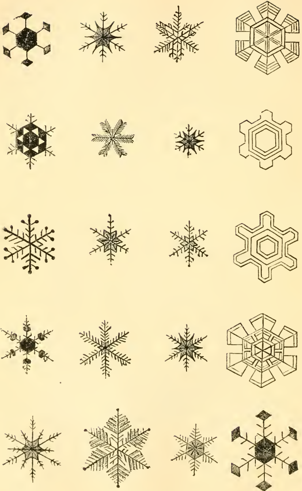
Fig. 94.— Snow Crystals.
