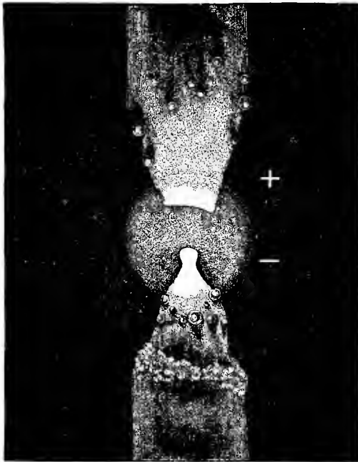
Voltaic Arc.
