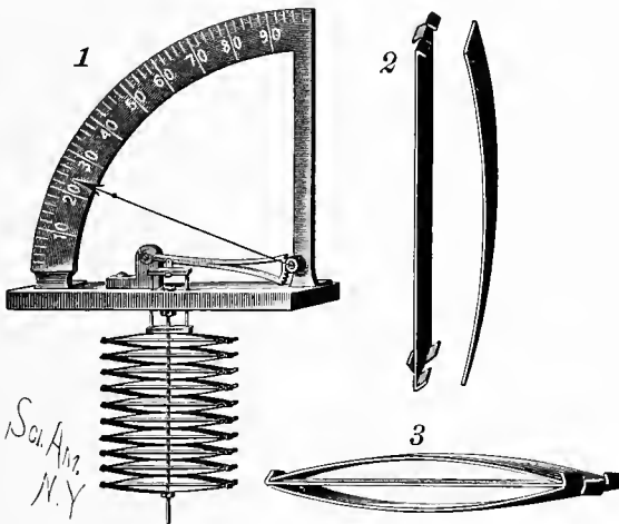
Thermostat.
