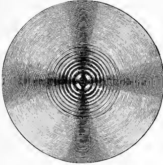
Calcite.
