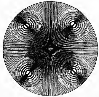
Aragonite Hemitrope.
