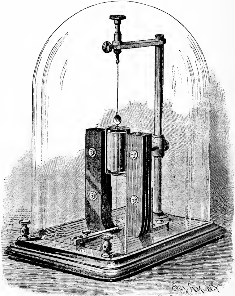
Deprez-D'Arsonval Galvanometer.
