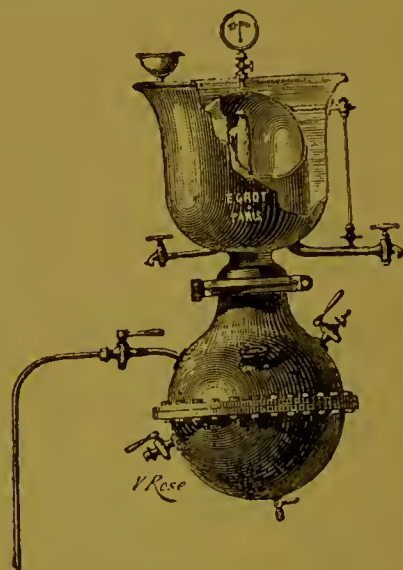
Appareils à concentrer dans le vide fonctionnant avec ou sans pompe dernier perfectionnement : Appareil à concentrer dans le vide, système EGROT et GENEVOIX.
